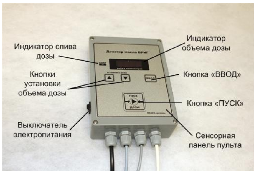
Рис 4: Пульт управления
