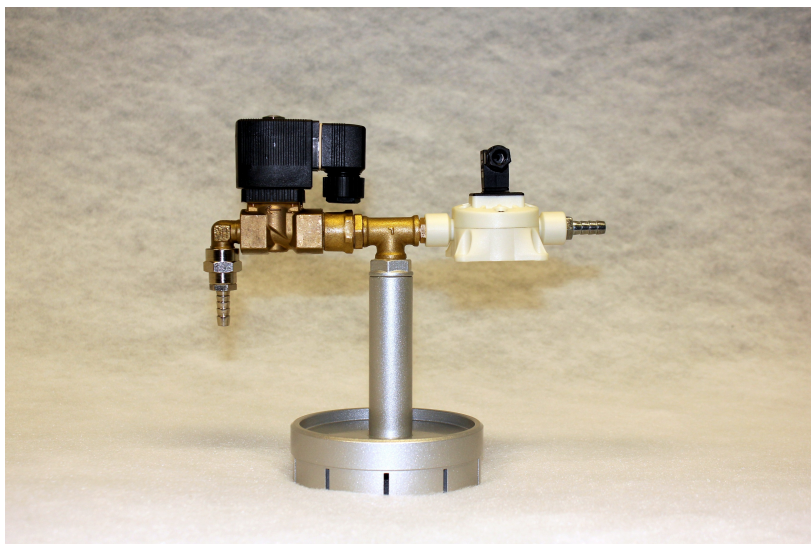
Рис 2: Дозирующее устройство
