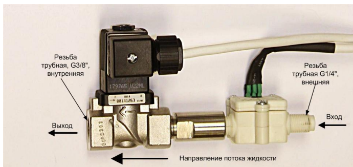
Рис 2: Подключение к магистрали
