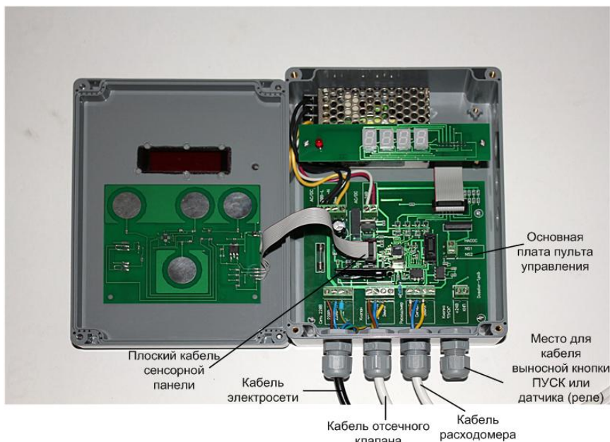
Рис 4: Пульт управления со снятой крышкой
