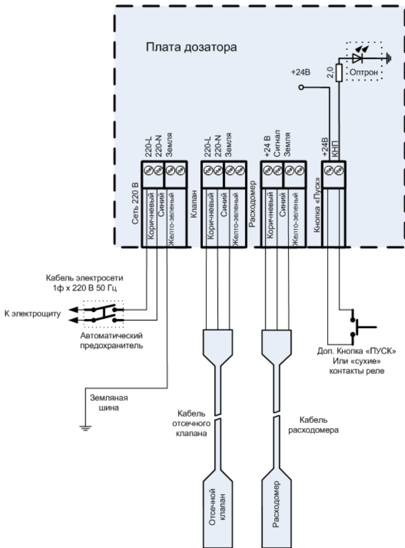
Рис 5: Монтажная схема дозатора
