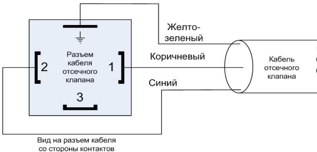
Рис 5: Подключение кабеля к отсечному клапану
