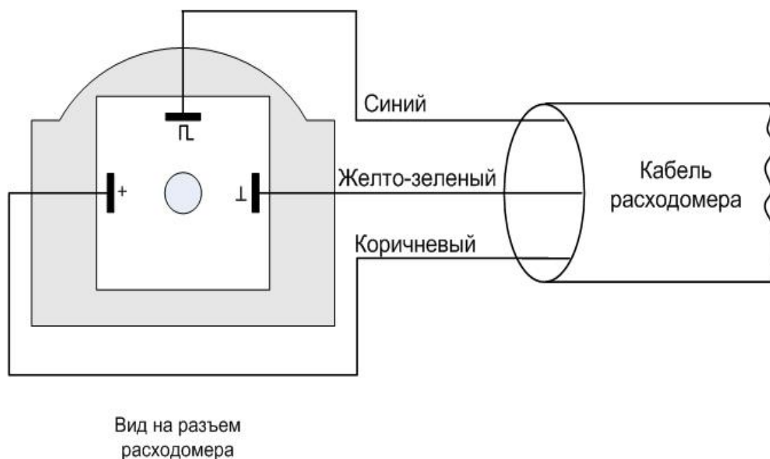
Рис 7: Подключение кабеля к расходомеру
