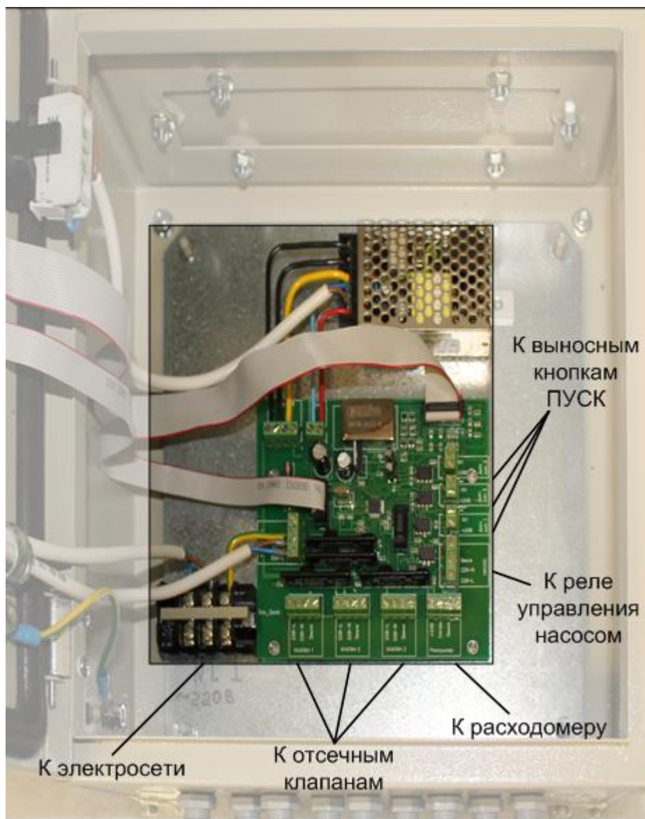
Рис 3: Пульт управления с открытой дверцей
