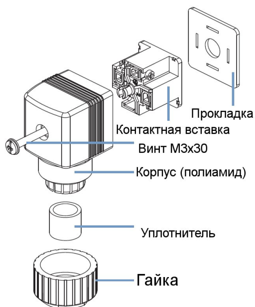
Рис 6: Разъем отсечного клапана
