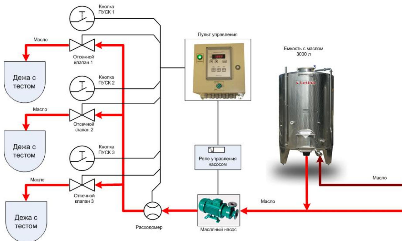
Рис 1: Структурная схема дозатора масла
